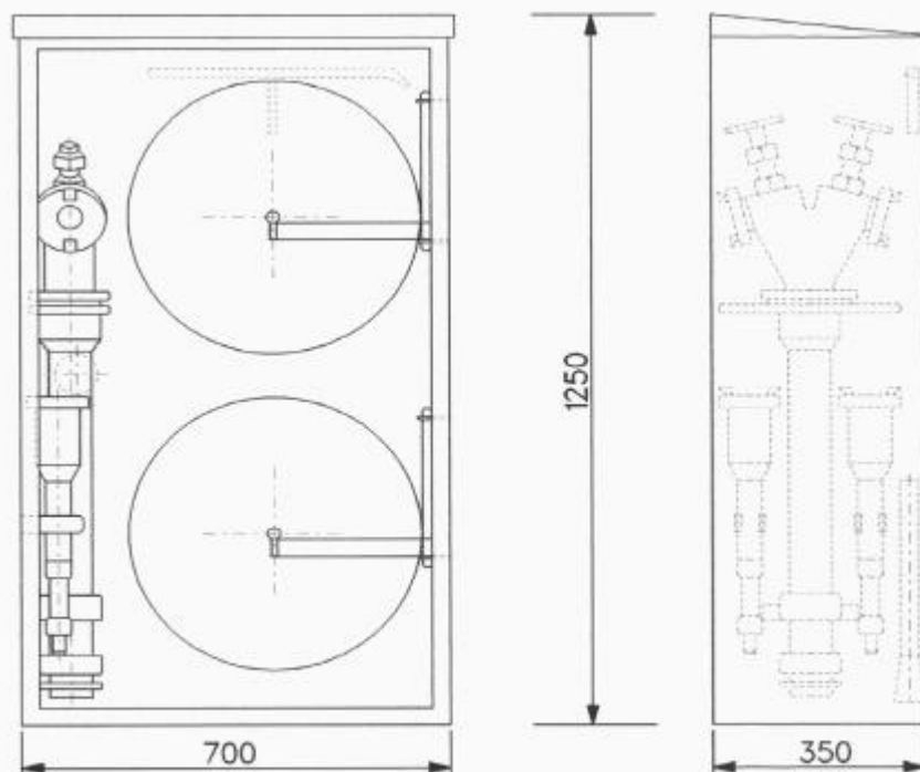
Ansicht ohne Tür gez.
